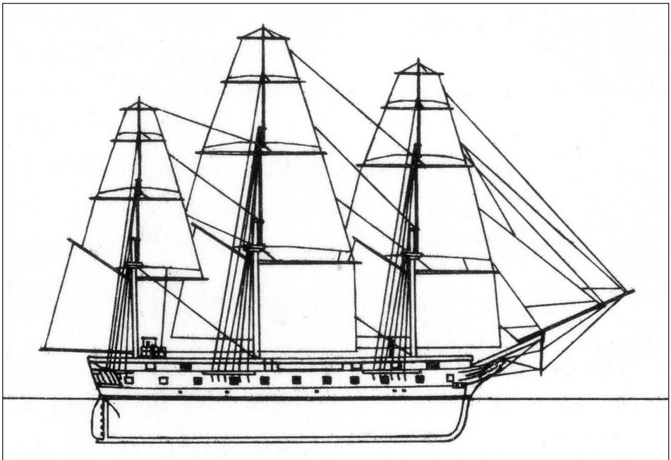
Abb. 7a–b Segelfregatte S.M.S. NIÖBE. (Aus: Wittmer [wie Anm. 66]). Unten: Skizze der NIÖBE (Aus: Gröner et al. [wie Anm. 38])
