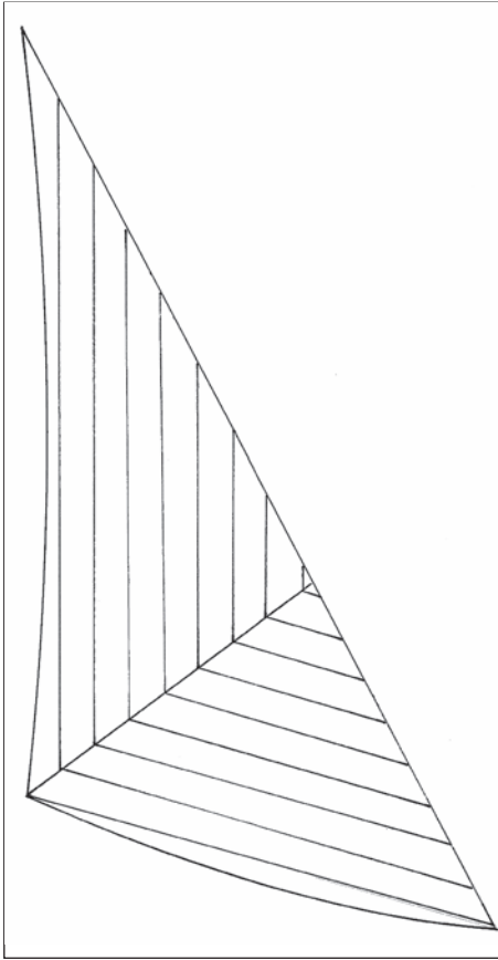
Abb. 8 Matthew Orrs Zuschnitt, bei dem sich die Tuchkleider parallel zur Achter- und Unterseite orientieren – und sich in einer winkelhälbierten Lasche treffen. (Zeichnung: Verf.)
