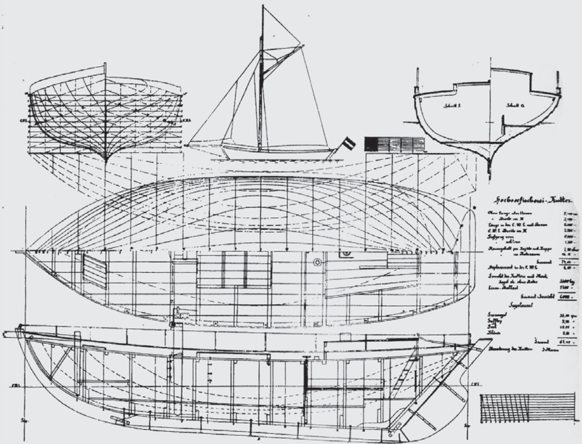
Abb. 14 Lachskutter. (Zeichnung: C. Engel, aus: Engel 1897)
