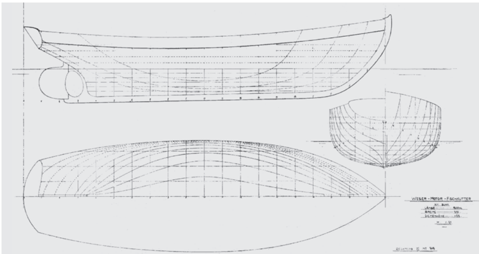
Abb. 77 Weser-Motor-Fischkutter mit Bün (Länge 12,00 m, Breite 3,70 m, Seitenhöhe 1,55 m). Zeichnung XII Nr. 242 im Maßstab 1:20, Lürssen Werft, 1919. (Bundesarchiv, Sign. R/8838-80)
