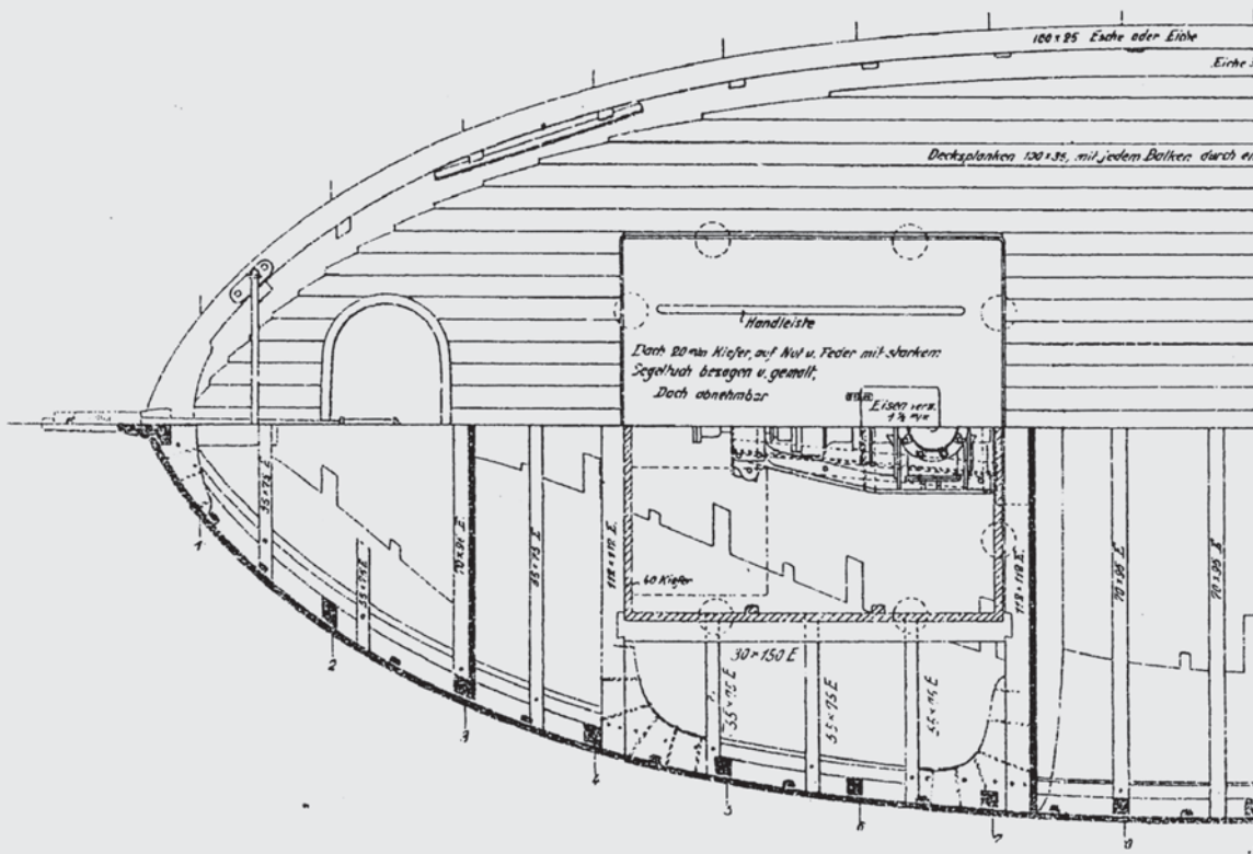
Abb. 59 Motorfischkutter, Typ Pommern. (Aus: Müller 1922)
