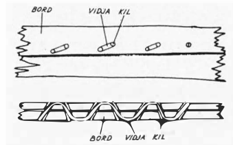
Abb. 7 Nähetechnik im Fund eines wahrscheinlich russischen genähten Bootes aus der Skeppargata in Stockholm.
