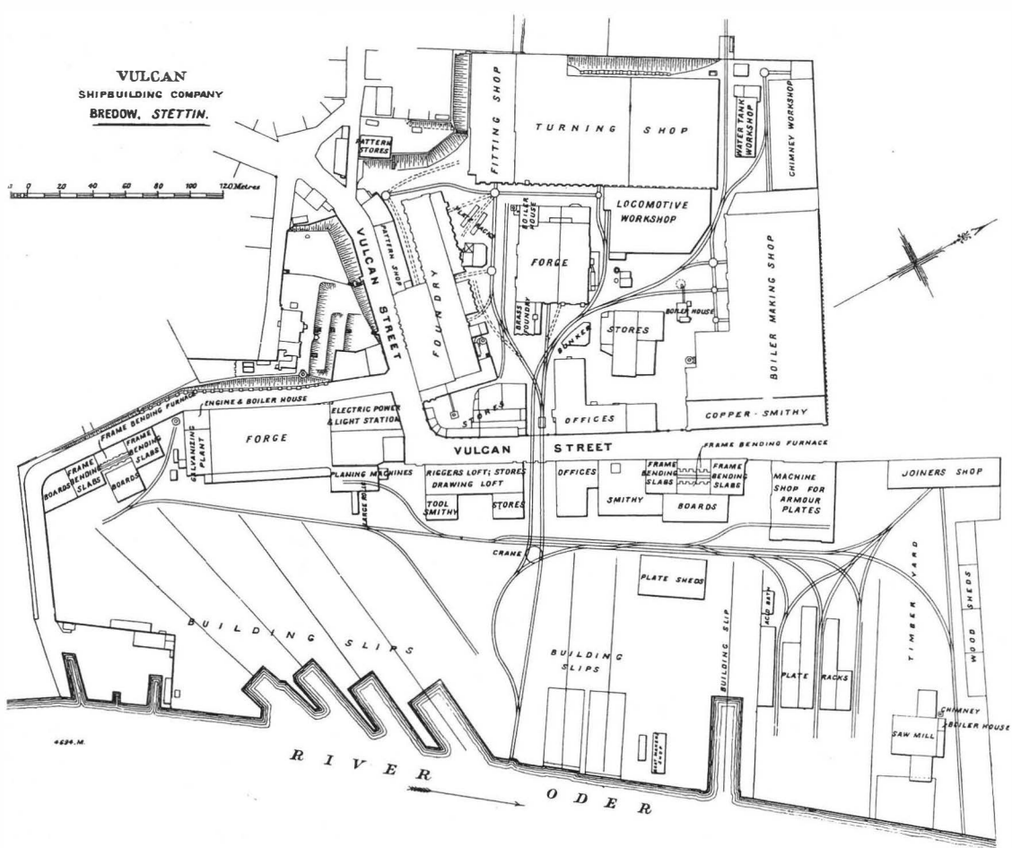
Abb. 2 Plan des Vulcan-Werkgeländes in Bredow, Stettin (aus: Stettiner Maschinenbau Actien-Gesellschaft »Vulcan«, 1899).
