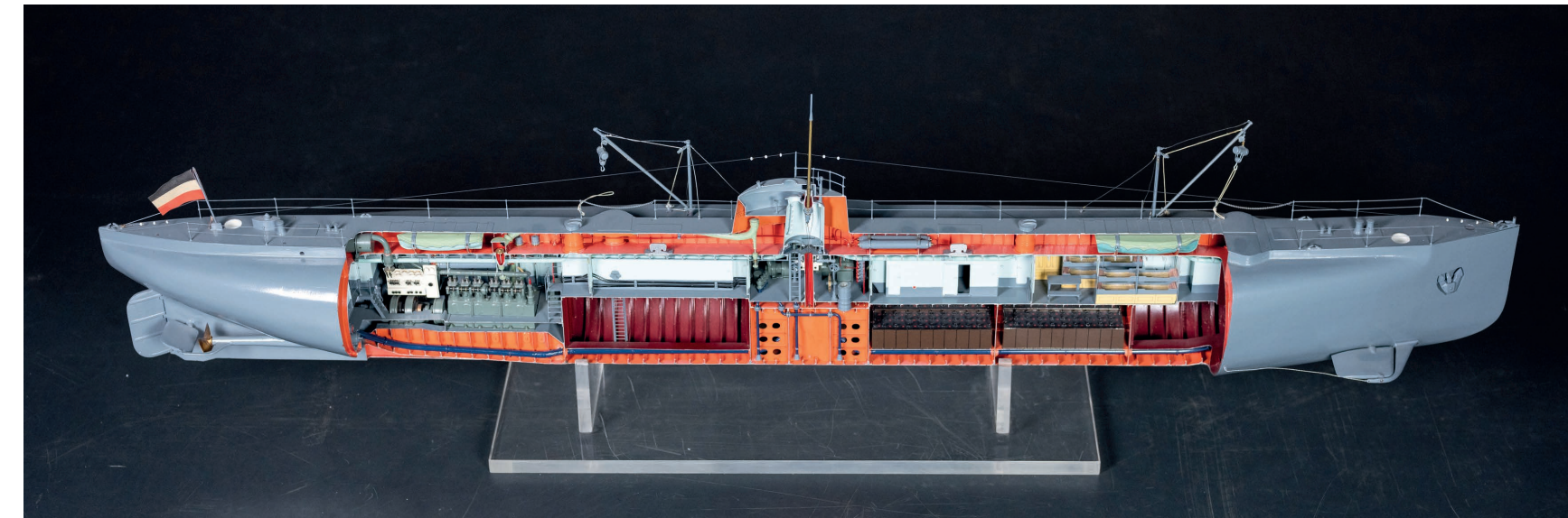
Modell des Handels-U-Bootes DEUTSCHLAND, teilweise als Schnittmodell gestaltet.
