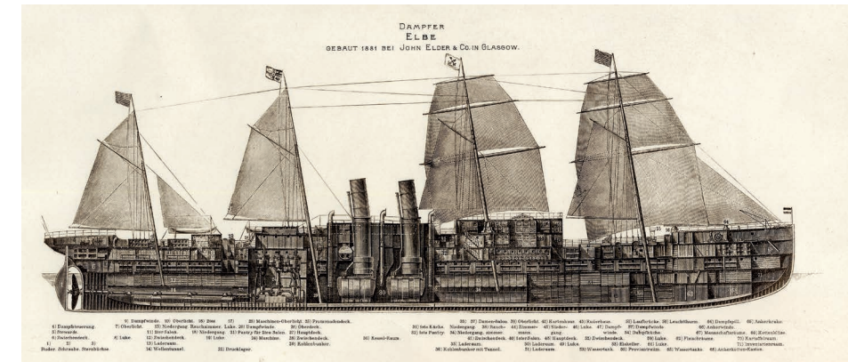
Zeitgenössischer Längsschnitt der ELBE, gebaut 1881.
